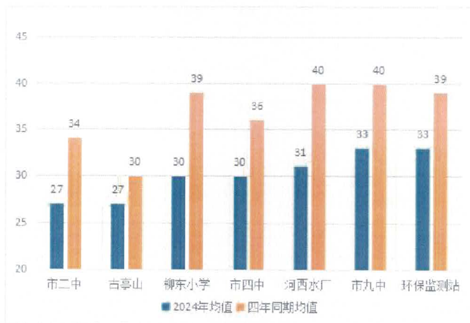
图 2 柳州市近四年来 1-4 月的 PM 2.5 浓度均值与本年度对比
