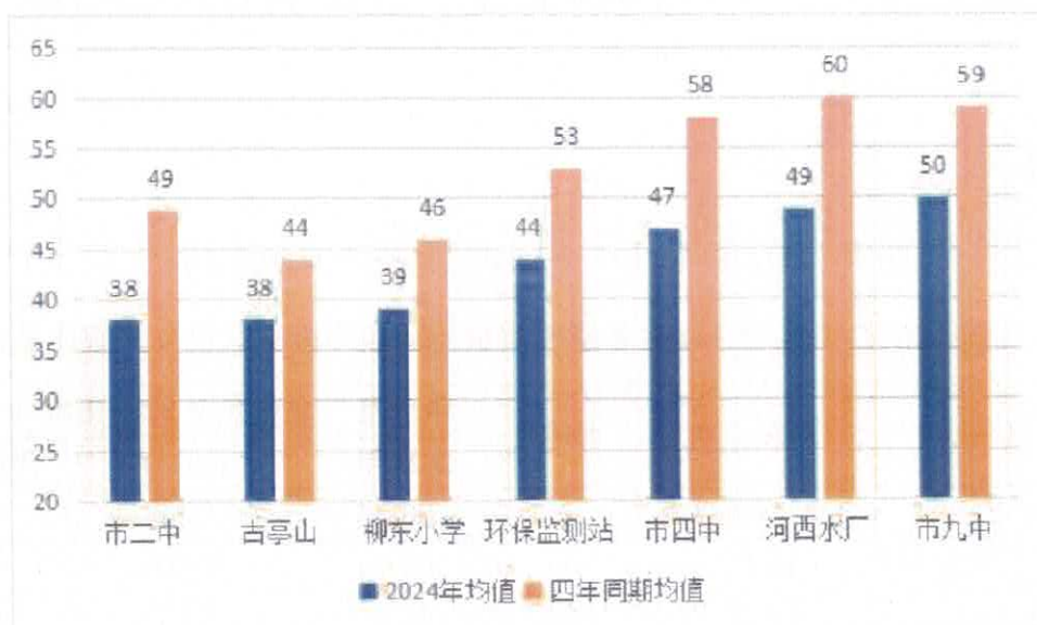
图 1 柳州市近四年来 1-4 月的 PM 10 浓度均值与本年度对比
