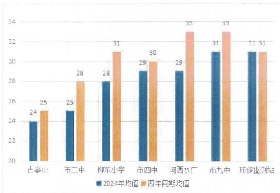
图 2 柳州市近四年来 1-5 月的 PM 2.5 浓度均值与本年度对比
