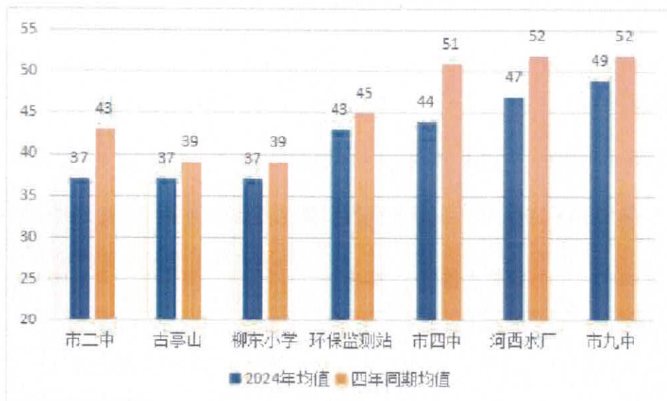
图 1 柳州市近四年来 1-5 月的 PM 10 浓度均值与本年度对比
